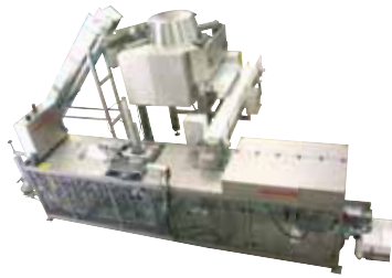
Pesage et ensachage de filets de poissons surgelés
